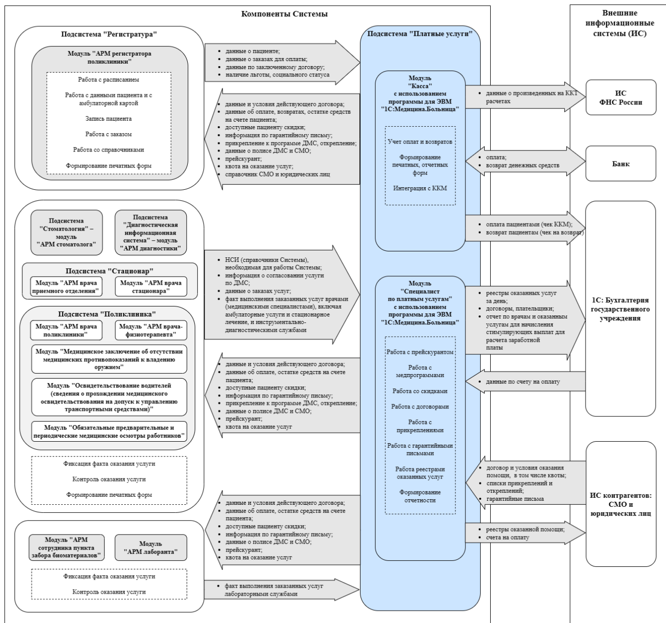
Рисунок А.3 – Схема взаимодействия компонентов (подсистем, модулей) Системы и сторонних систем
